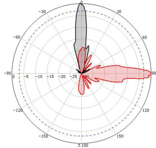
V-Pol@3500MHz
