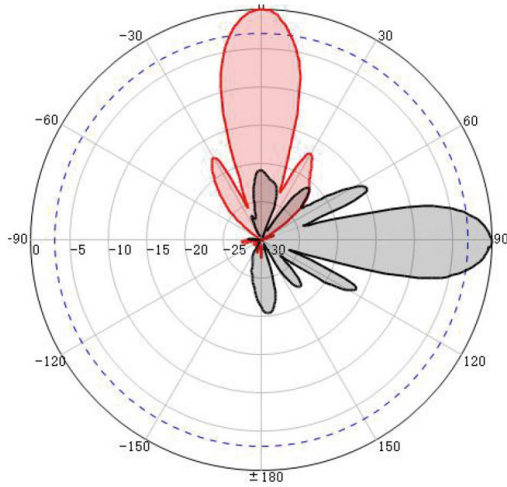
H-Pol@1710MHz
