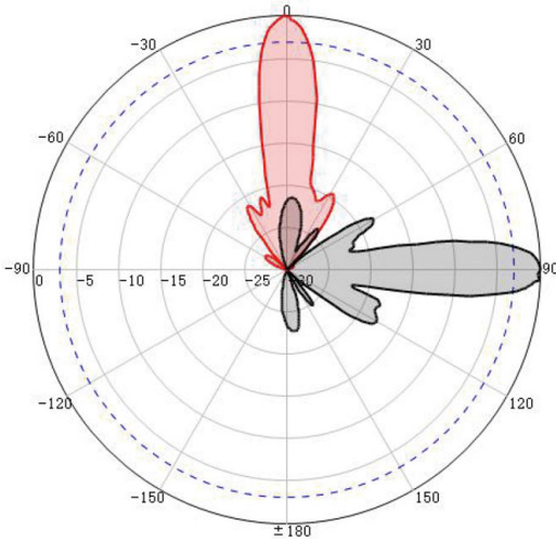
H-Pol@2700MHz
