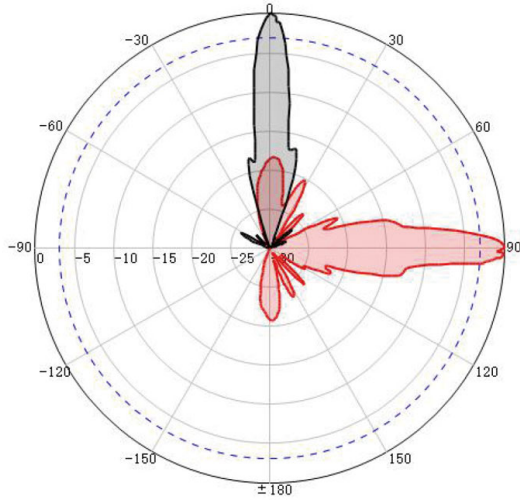
H-Pol@3500MHz
