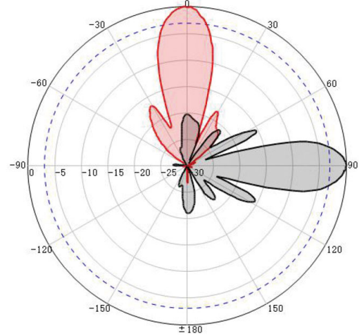
V-Pol@1710MHz
