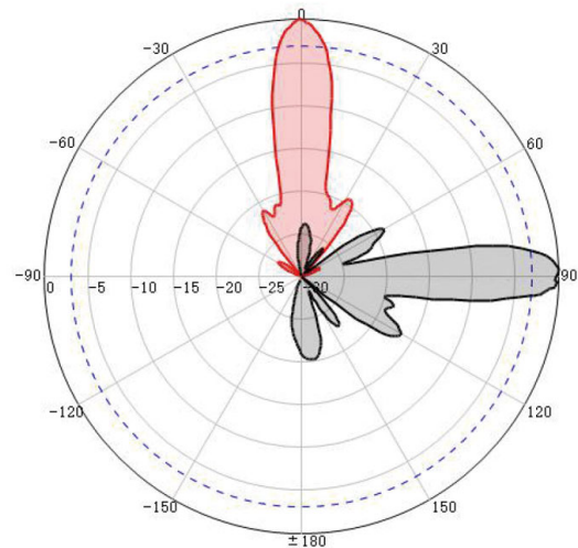
V-Pol@2700MHz
